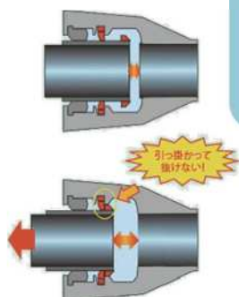
耐震継手管の構造（イメージ図）
